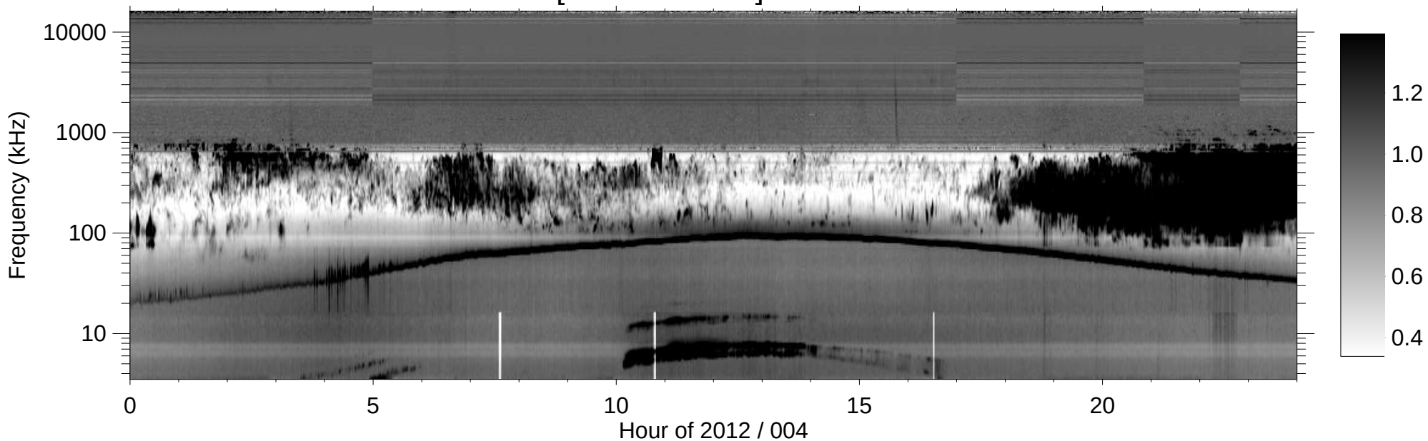
RPWS [ABCH1H2/Ex] (-B) 2012/01/04
