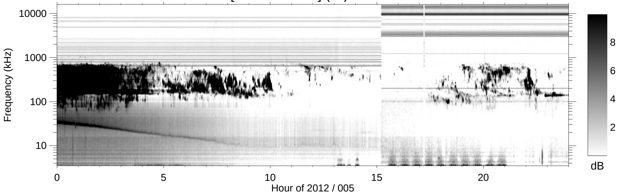
RPWS [ABCH1H2/Ex] (-B) 2012/01/05
