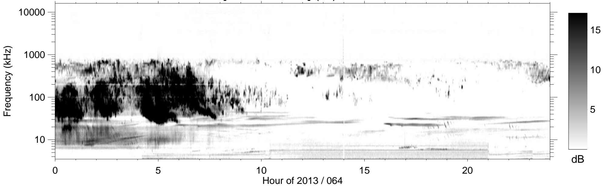
RPWS [ABCH1H2/Ex] (-B) 2013/03/05
