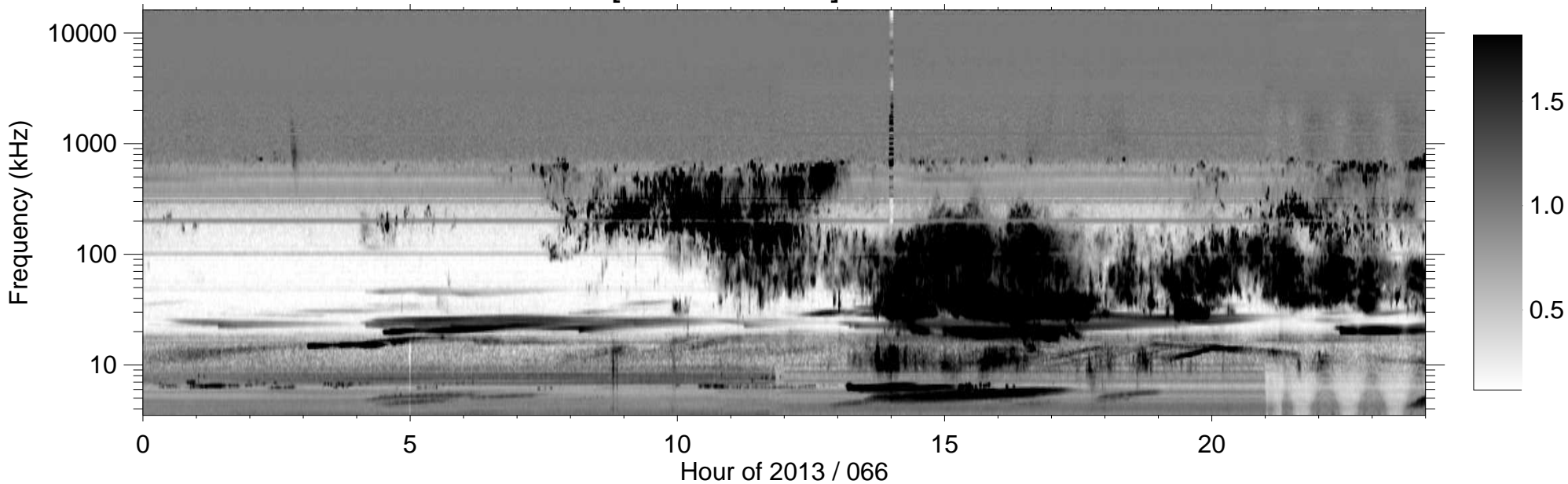
RPWS [ABCH1H2/Ex] (-B) 2013/03/07
