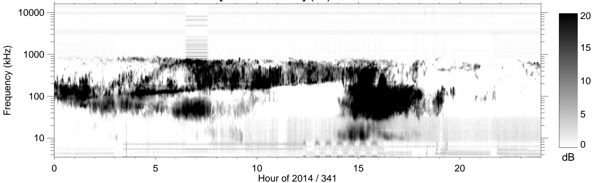
RPWS [ABCH1H2/Ex] (-B) 2014/12/07
