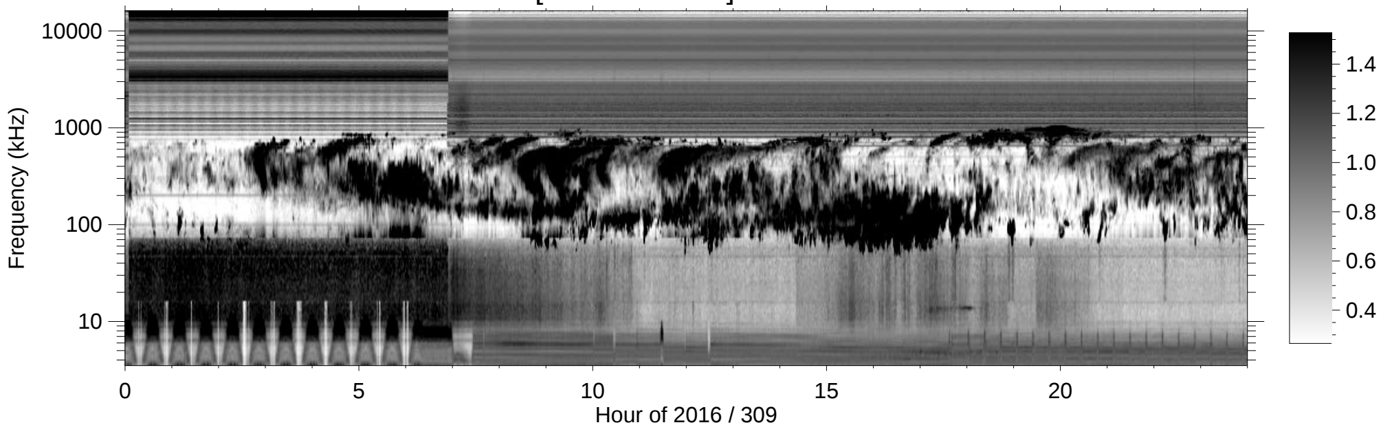
RPWS [ABCH1H2/Ex] (-B) 2016/11/04
